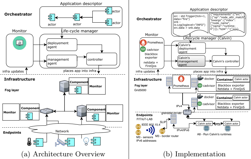
Fig. 1: FogIoT Orchestrator
